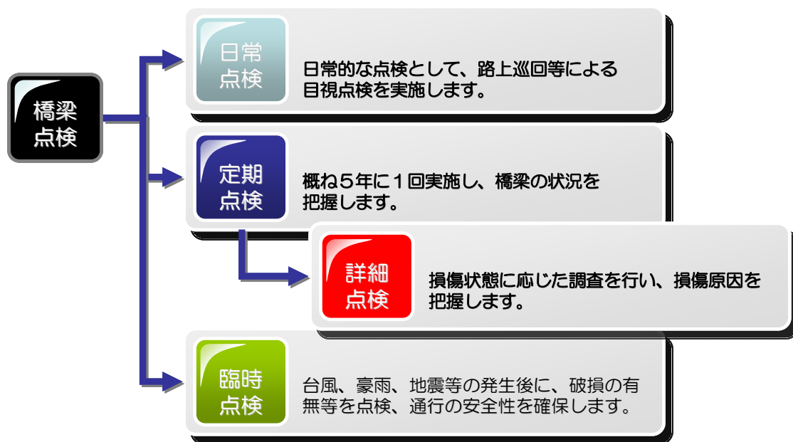
図2 橋梁点検フロー
